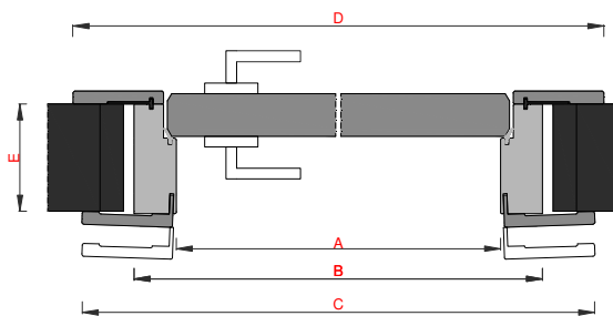
SEZIONE ORIZZONTALE
